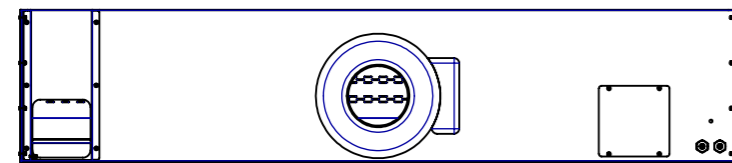
SECTION A-A
